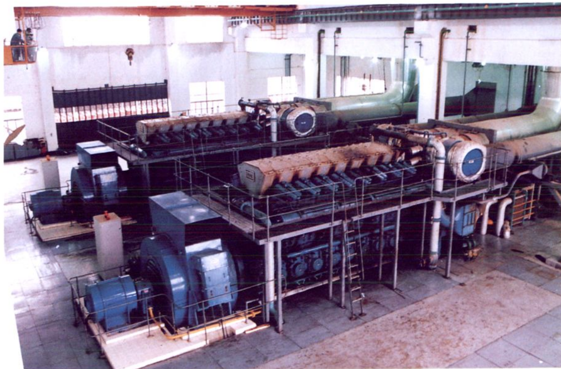
清远市建北发电厂装机容量 2 \times 1.13 万千瓦(1991年建成)
