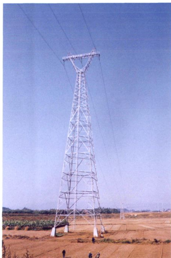
清远市最高的铁塔220千伏清阳乙线 北江河大跨越塔(BK-78塔高82.5米, 2000年5月送电)
