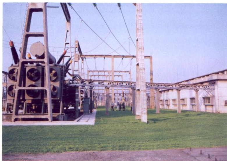
220千伏英德变电站 (1993年12月投产)
