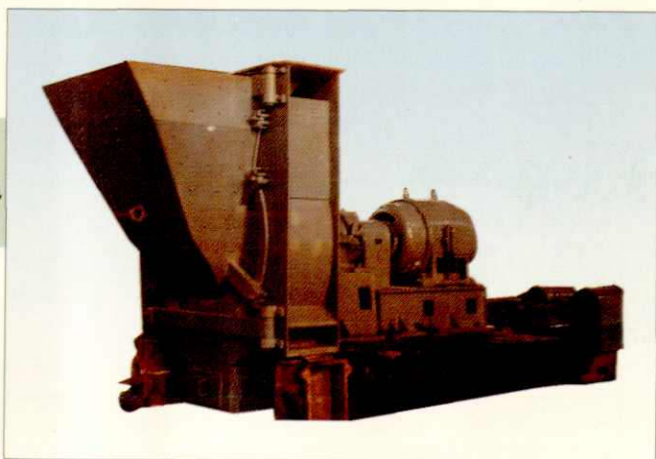
风扇磨煤机
