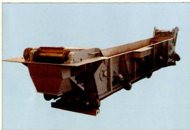
刮板捞渣机
