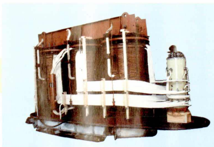
中性点有载调压变压器
