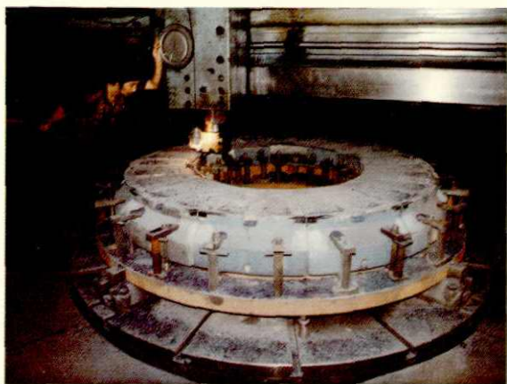
金工车间加工MPS中速磨衬瓦
