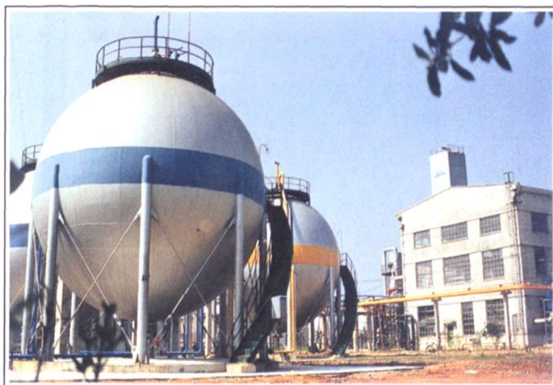
具有 80 年代国际先进水平的 6000 米 3 /时制氧站。
