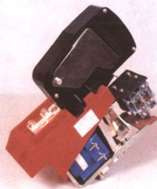
CCZ38-1250/10直流接触器
