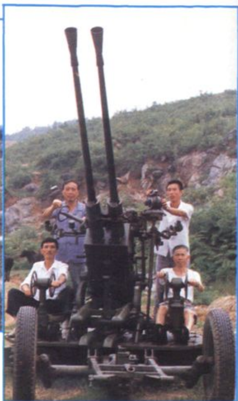
△高炮人工降雨作业
