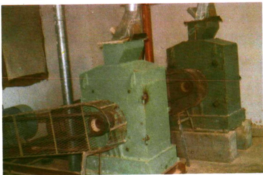
城关米厂大米车间加工设备去石机
