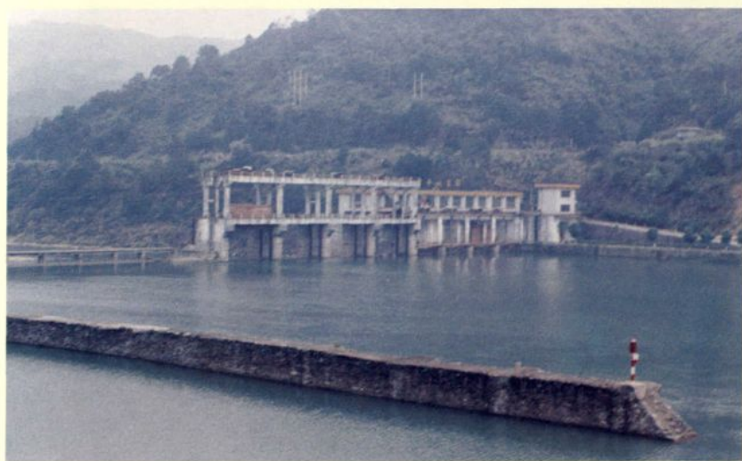
◀ 英德市黄茅峡电站，装机容量5960千瓦（1991年建成）
