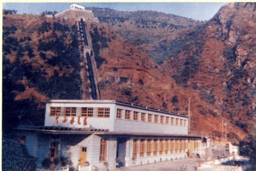
◀ 英德市大镇空子水电站，装机容量 3 \times 1250 千瓦（1979年建成）
