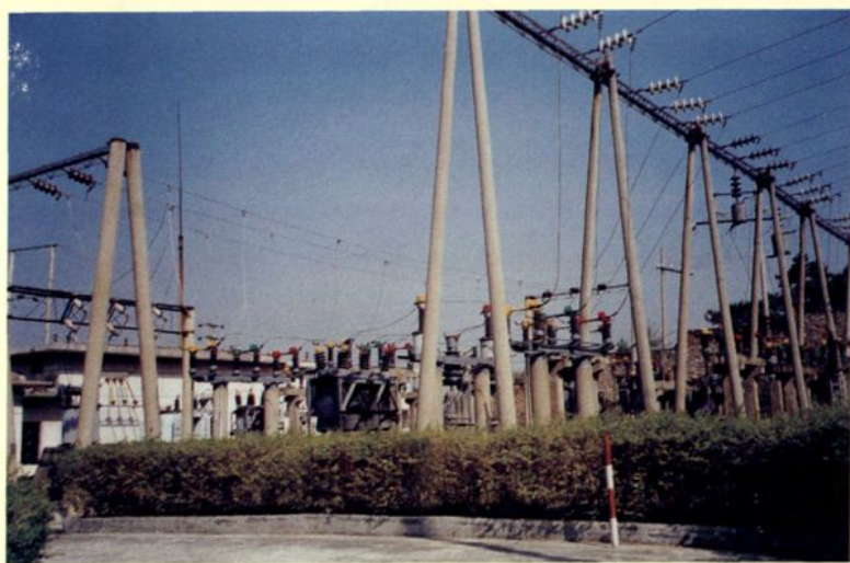
◀ 35千伏寺前变电站（1986年建成）
