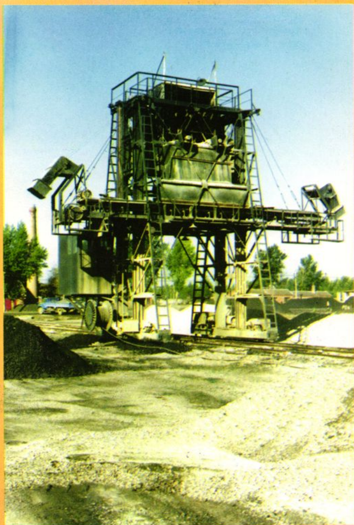
1980年10月投入使用的二货场70型散卸机
