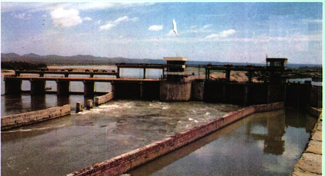
▼ 永安发电所进水枢纽
