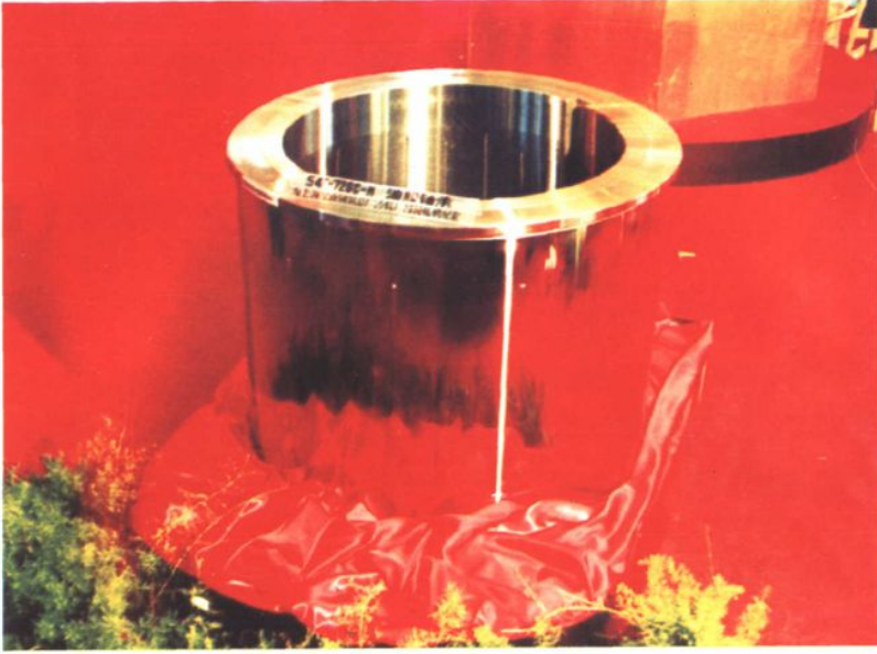
为上海宝钢生产的54"-720C-H油膜轴承
