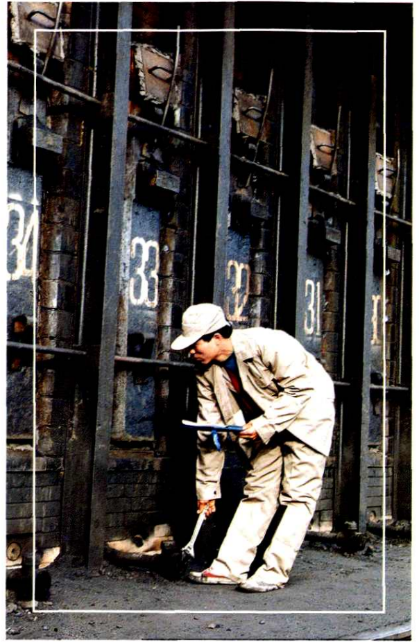
机焦炉
