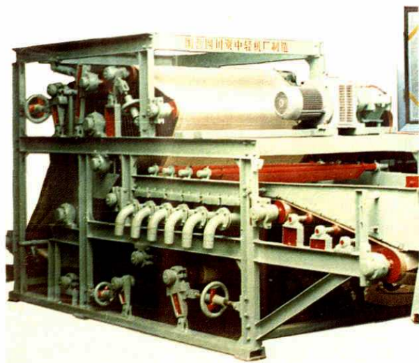
△轻机厂双网压滤真空洗浆机
