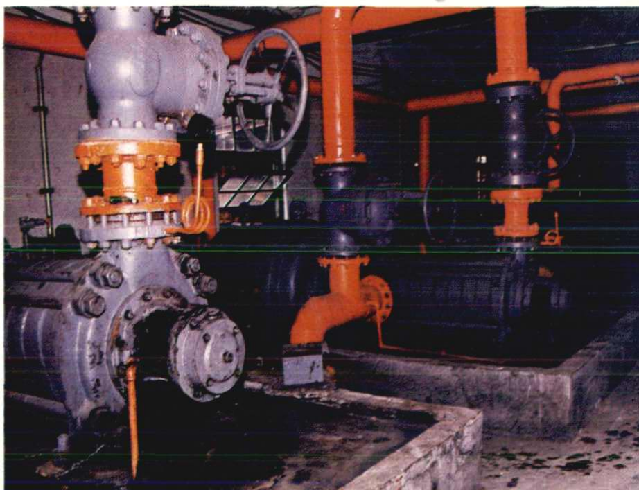
• 可串的高压泵
