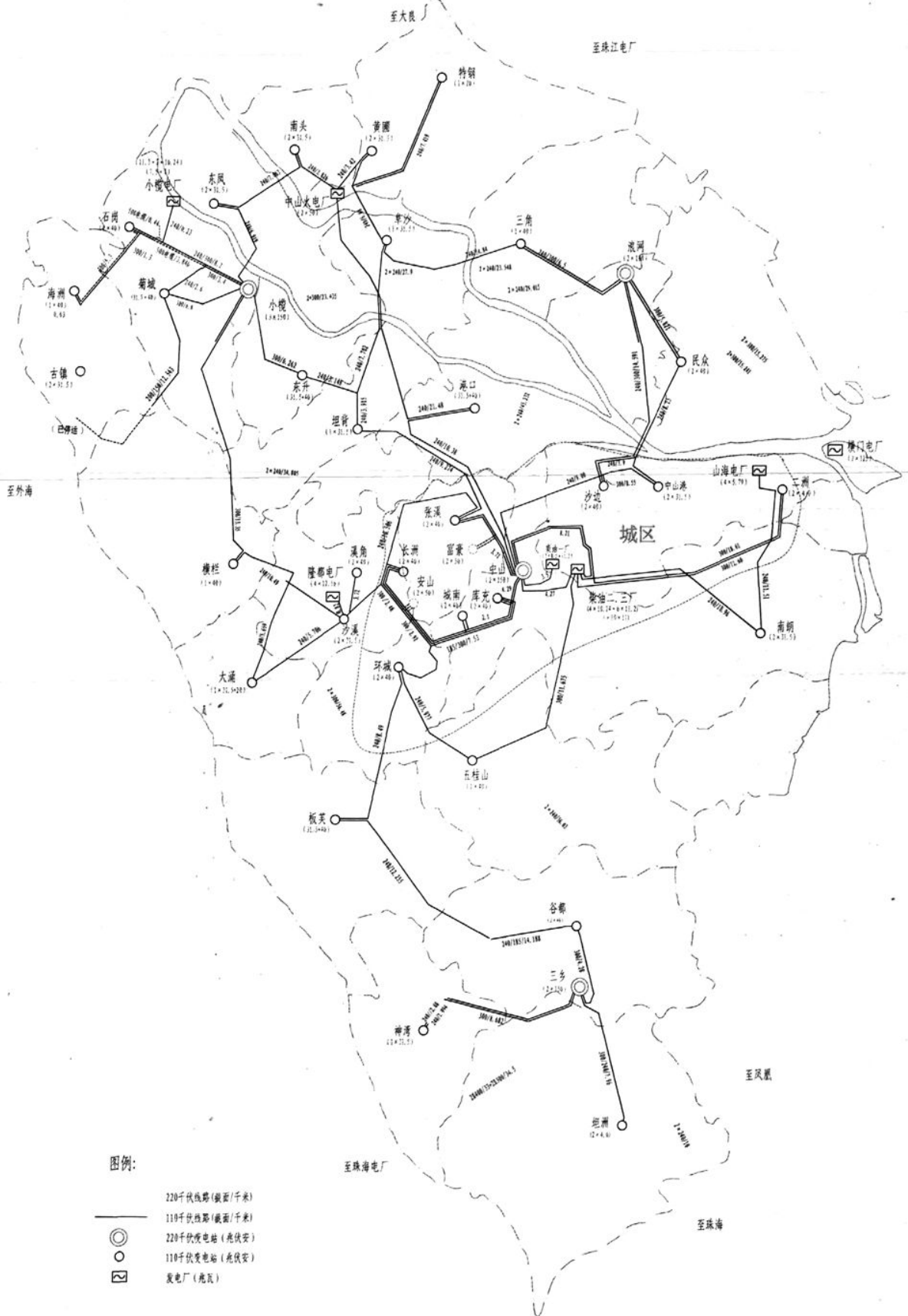
2000年中山电网地理接线图
