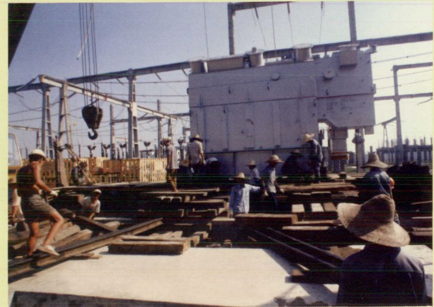
▲ 小榄站主变压器安装
