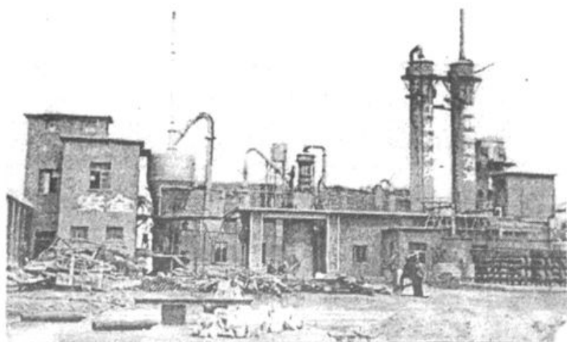
建厂初期生产厂区 (图为年产五千吨 硫酸生产装置)
