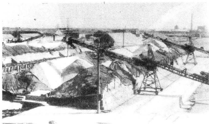
原盐集坨机械化
