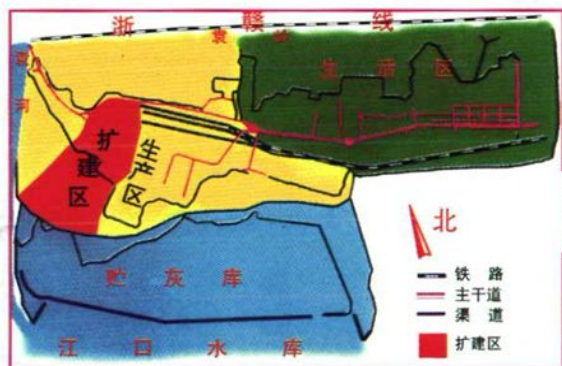
分宜发电厂地理位置图、厂区平面图
