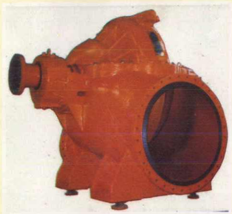
兰州水泵厂1200S系列单级双吸离心泵
