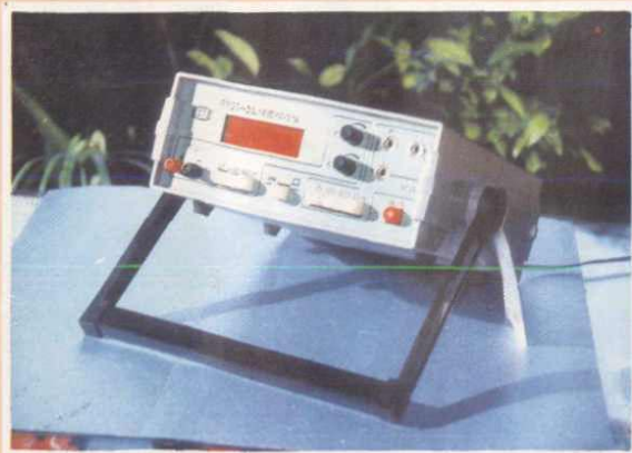
天水长城精密电表厂PF27-3精密校准仪
