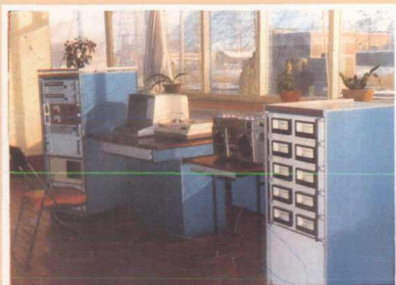
天水红山试验机厂双台面微机轨道衡控制室
