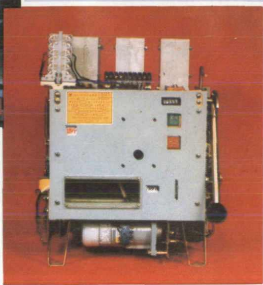
天水长城低压电器厂DW15系列框架式万能式空气断路器
