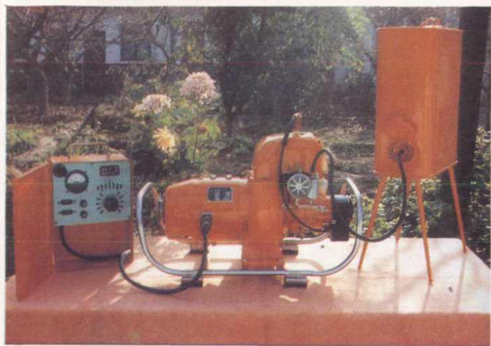
甘肃省电影机械厂 1GF4 型汽油发动发电机
