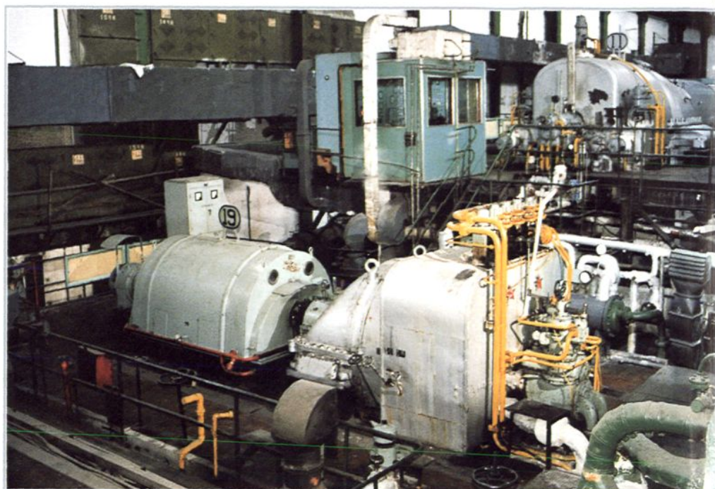
1958年自行安装的国产6000千瓦汽轮发电机组
