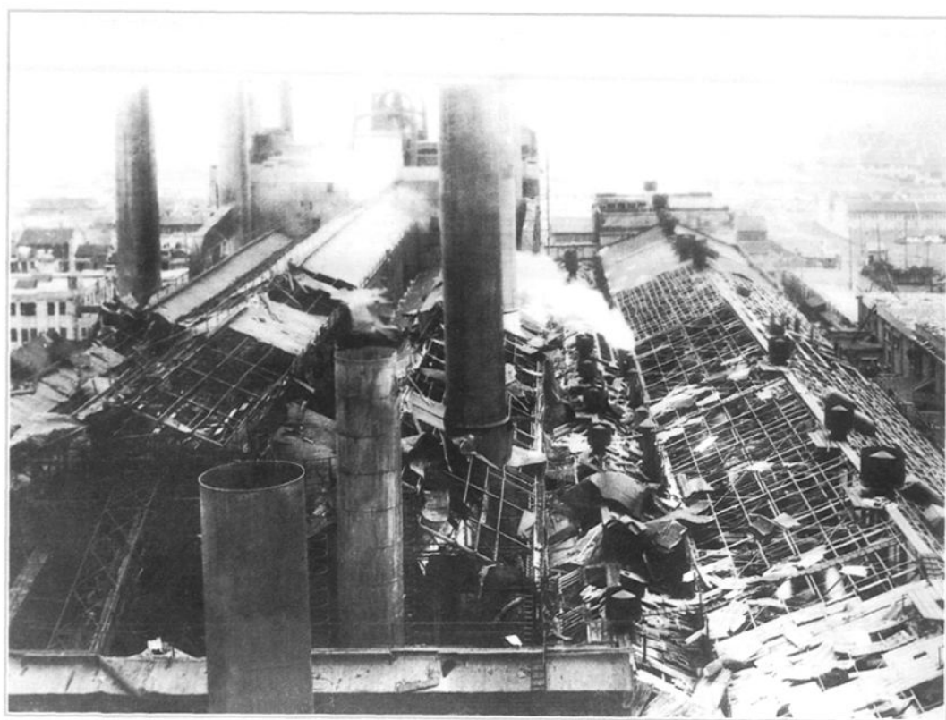
1950年“二·六”轰炸后，二、三号锅炉房及汽机房屋面受损情况
