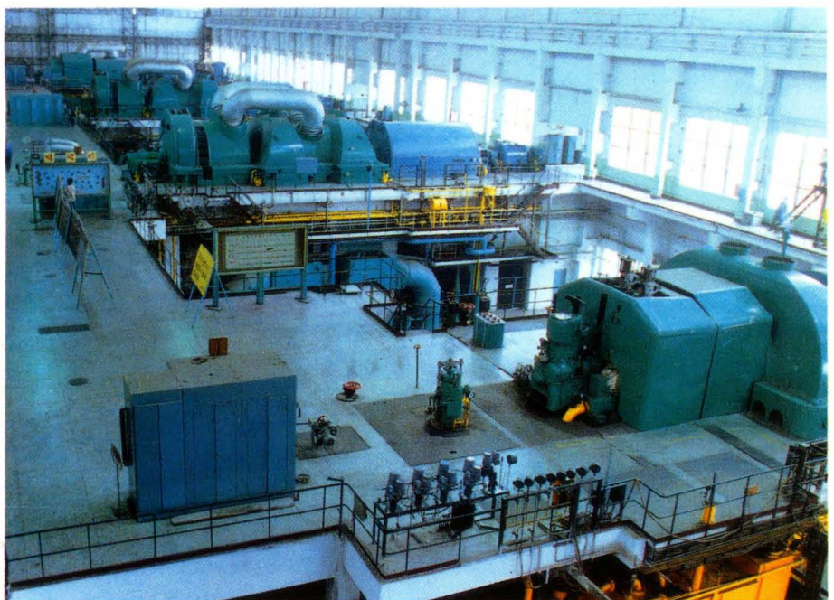
汽机车间 (1-4号机组)
