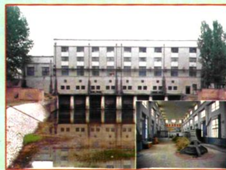
金堤河张庄电排站机房及厂房机组 (1975~1981)
