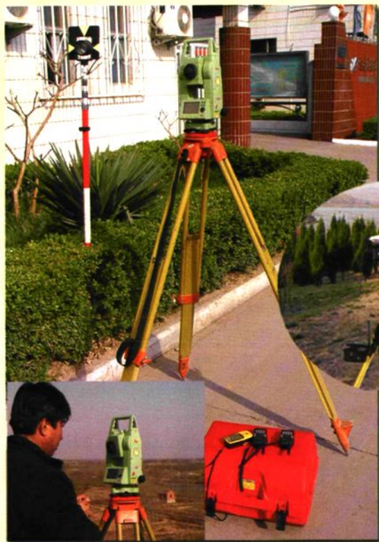
先进的测量设备—GPS、全站仪
