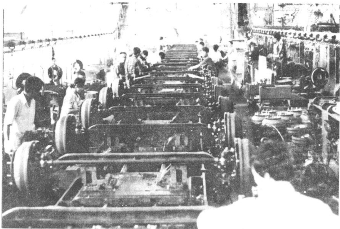
五吨车前桥装配线
