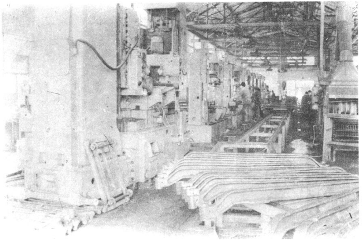
五吨车前梁生产线
