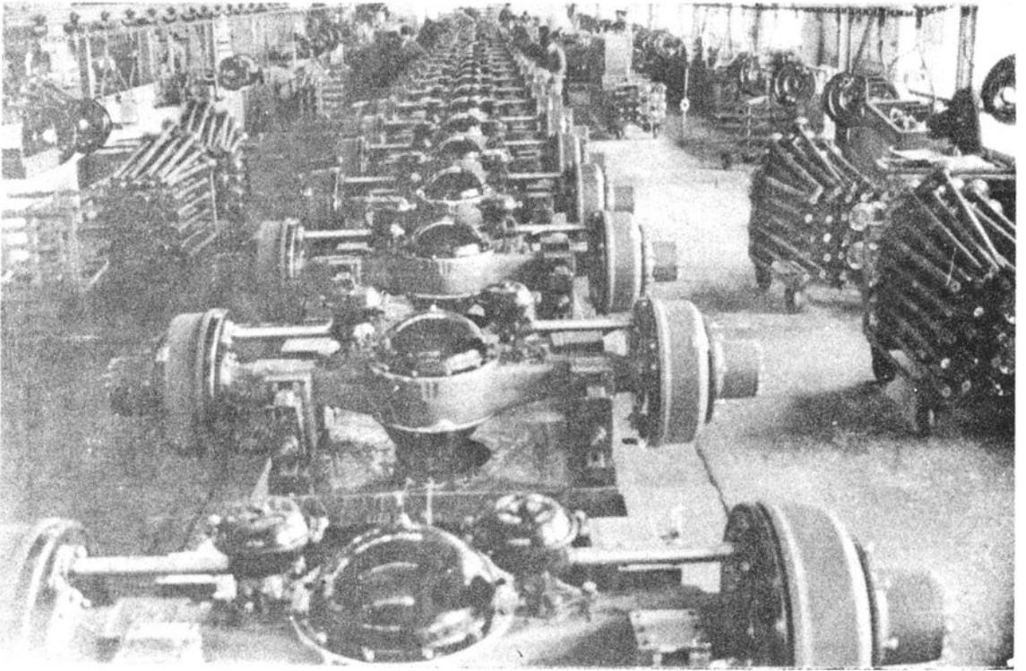
五吨车后桥装配线
