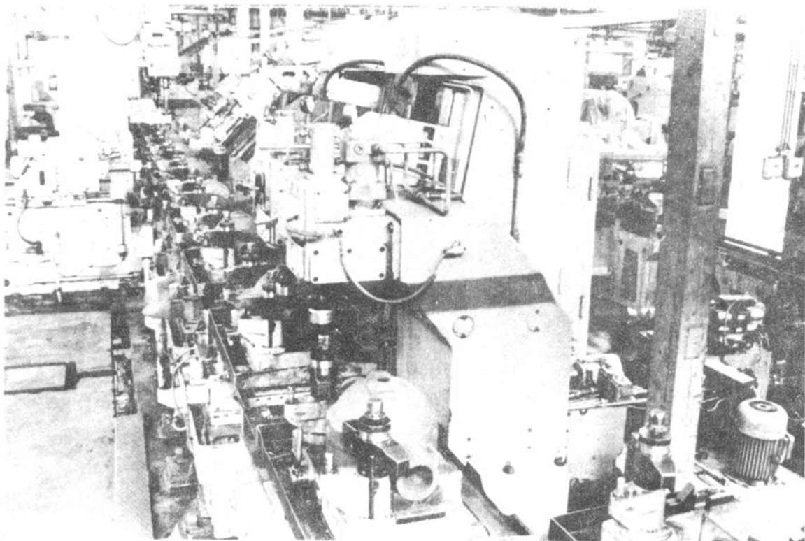
二吨半越野车桥壳自动线
