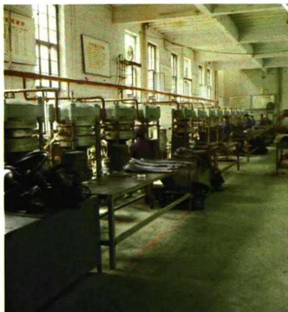
垫带硫化工艺
