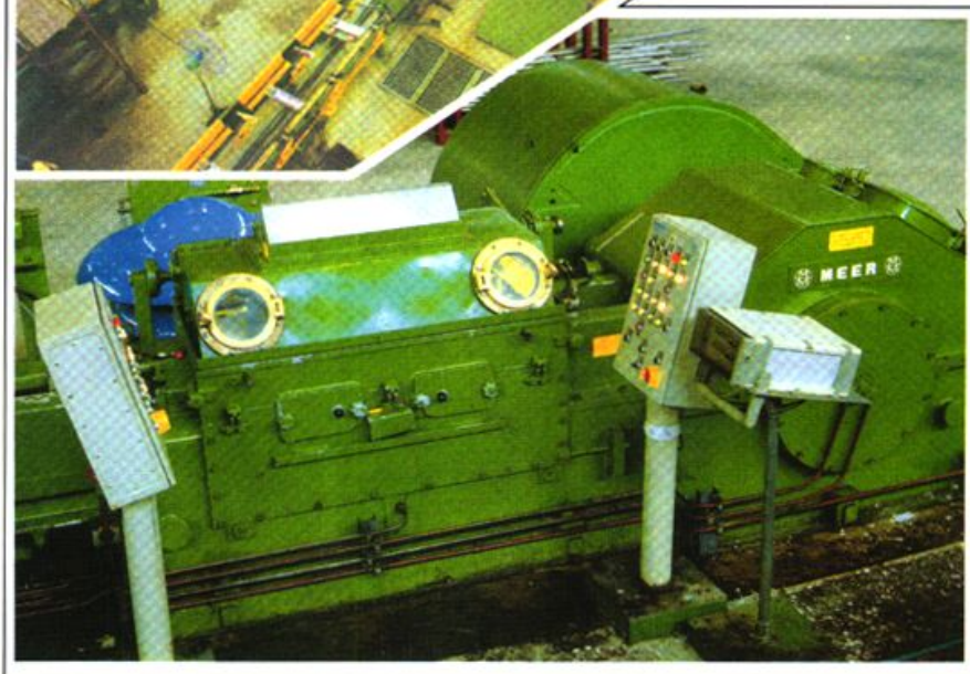
● 长钢从德国引进的冷轧机
