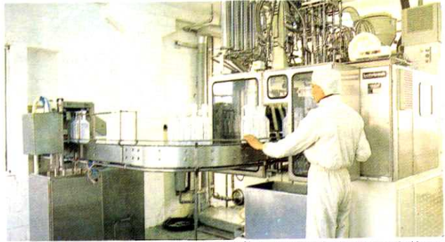
上海长征制药厂塑瓶输液制瓶灌装机
