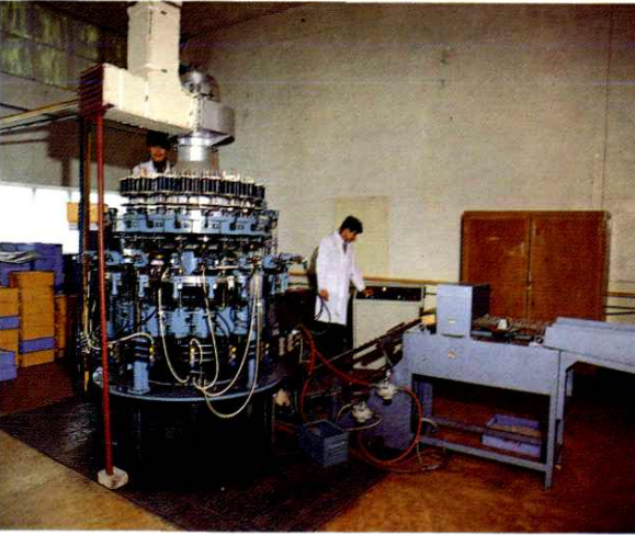
上海医用仪表厂日产3万支体温计的主要 设备
