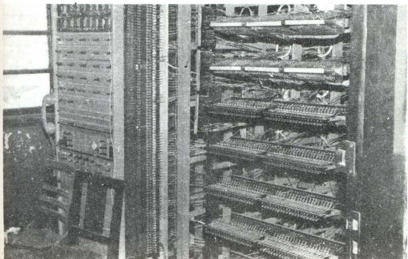
环十路载波机（殷波 摄）
