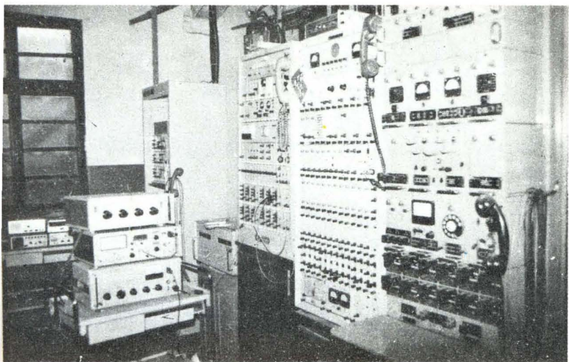
12路载波机（殷波 摄）
