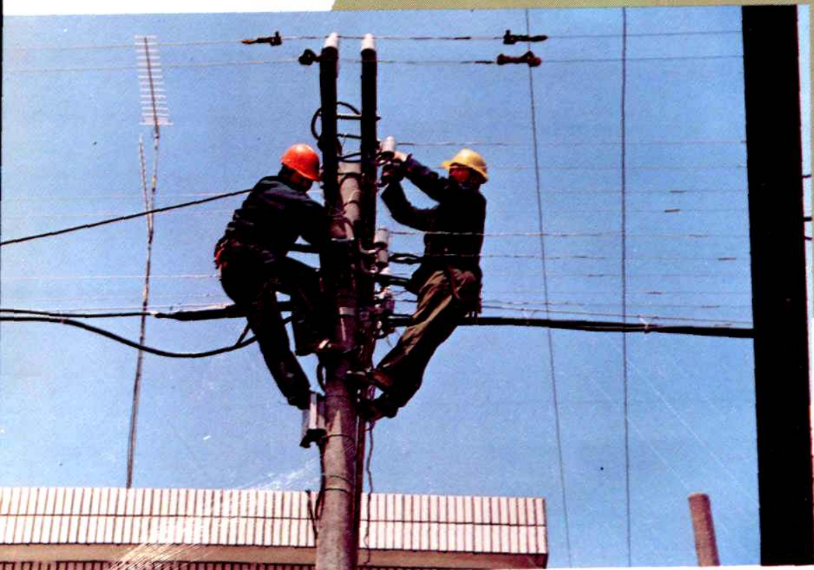
线务员在杆上作业
