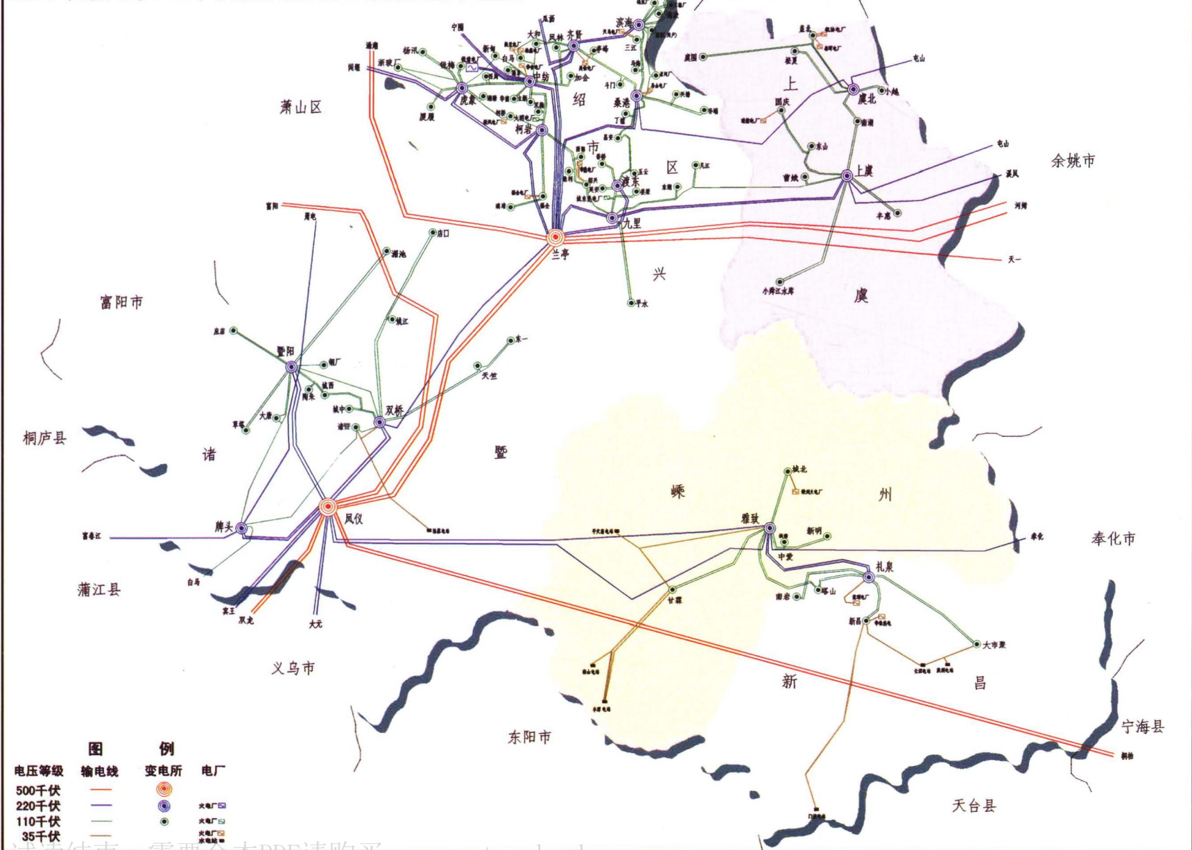
2005年绍兴市110千伏及以上电网地理接线示意图
