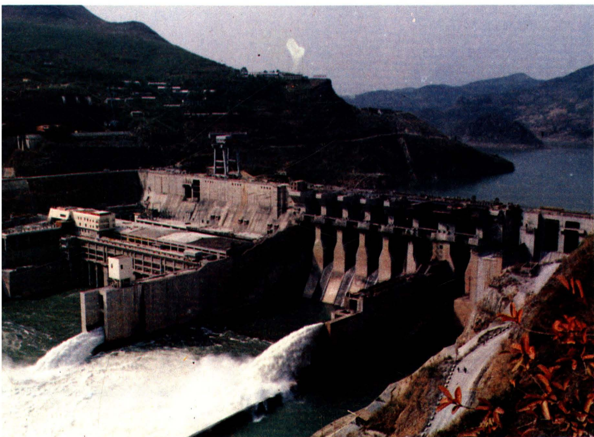
红水河岩滩水电站(121万千瓦) 罗安诚摄
