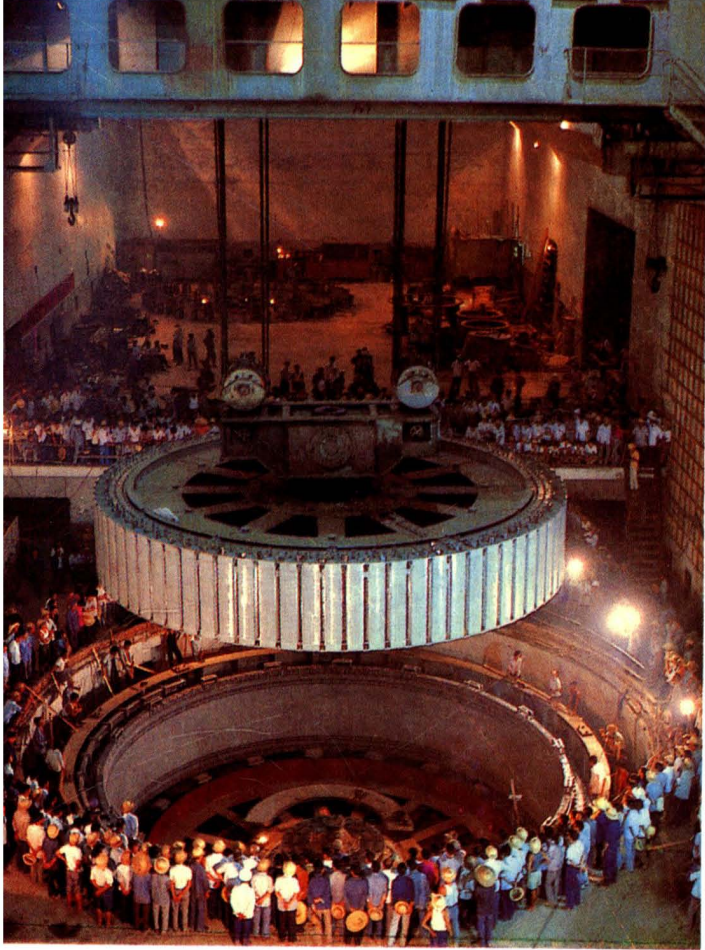
大化水电站1号发电机转子吊装 孙以宏摄
