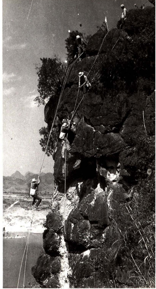
洛东水电站施工中处理险坡危石 谢庭滋提供
