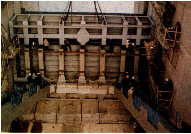
岩滩水电站溢流坝15×22.5米弧形闸门在吊装
