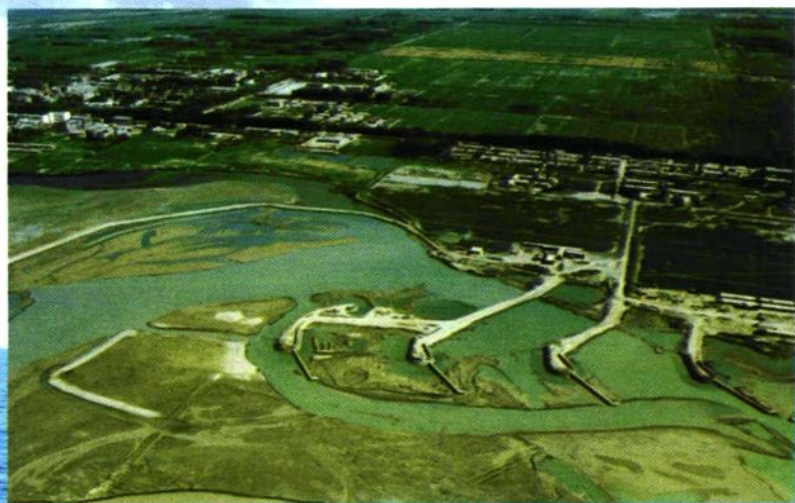
►塔里木河护岸 工程，有效地抵御 了河水对农田的危 害
