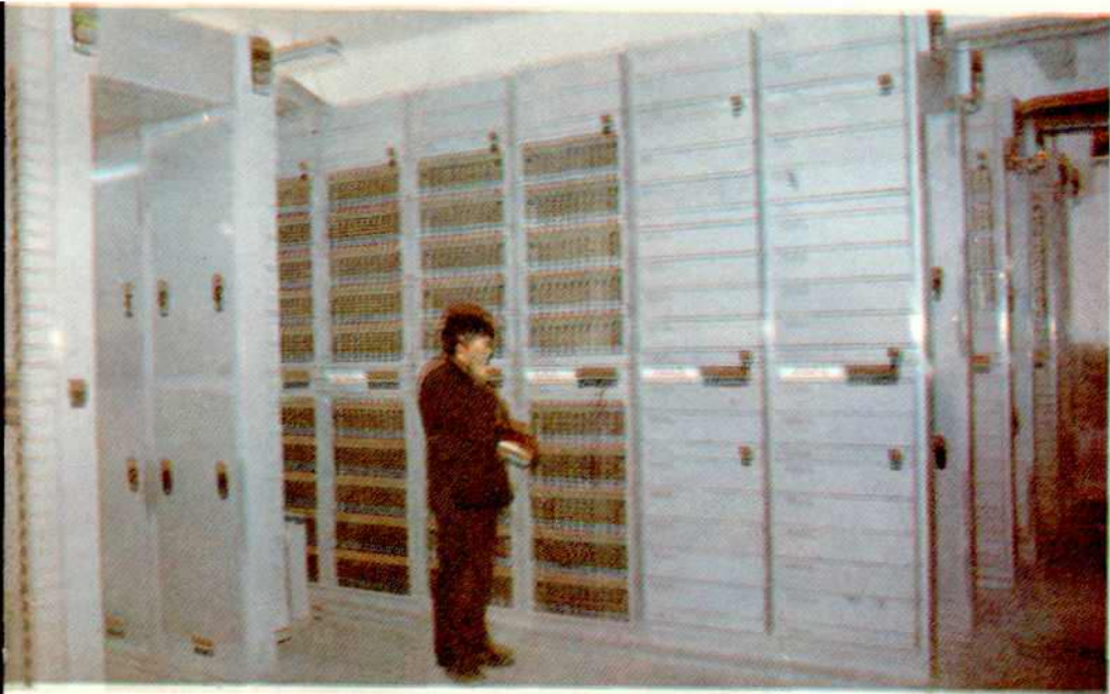
上：上海产 HJ—921A 型纵横制自 动电话交换 机2000门。
