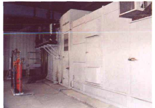
由公司安装调试的克拉玛依电厂 3.4 万千瓦燃汽轮发电机组
