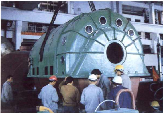
红雁池电厂 10 万千瓦机组汽轮机静子就位
