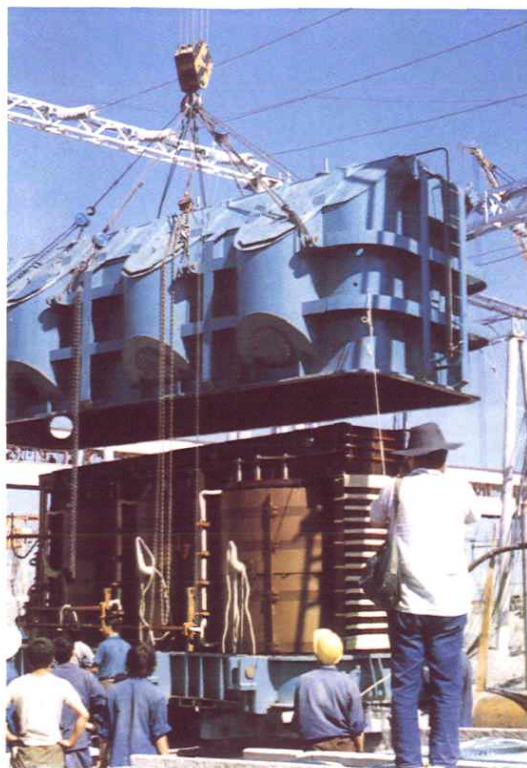
玛纳斯电厂 10 万千瓦机组主变压器安装
