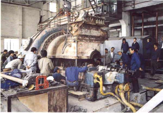
拜城电厂 1.2 万千瓦机组汽轮机扣大盖
