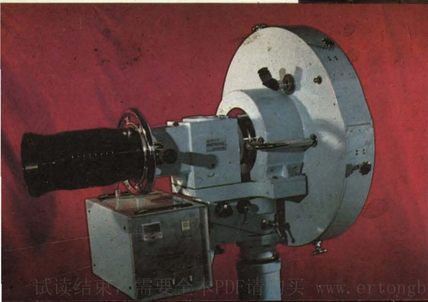
西安光机研究所研制的ZDF-180型转镜等待幅高速摄影机（李佑国摄）
