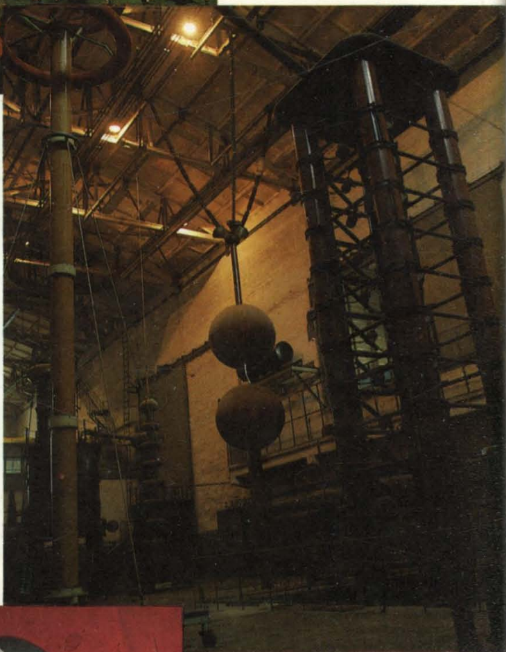
西安电力机械制造公司所属西安高压电器研究所高压试验厅之一
