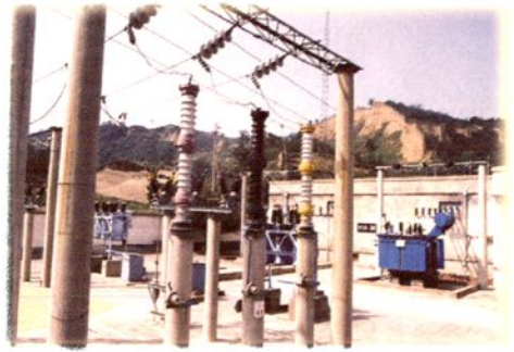
△ 岭上35千伏变电站
