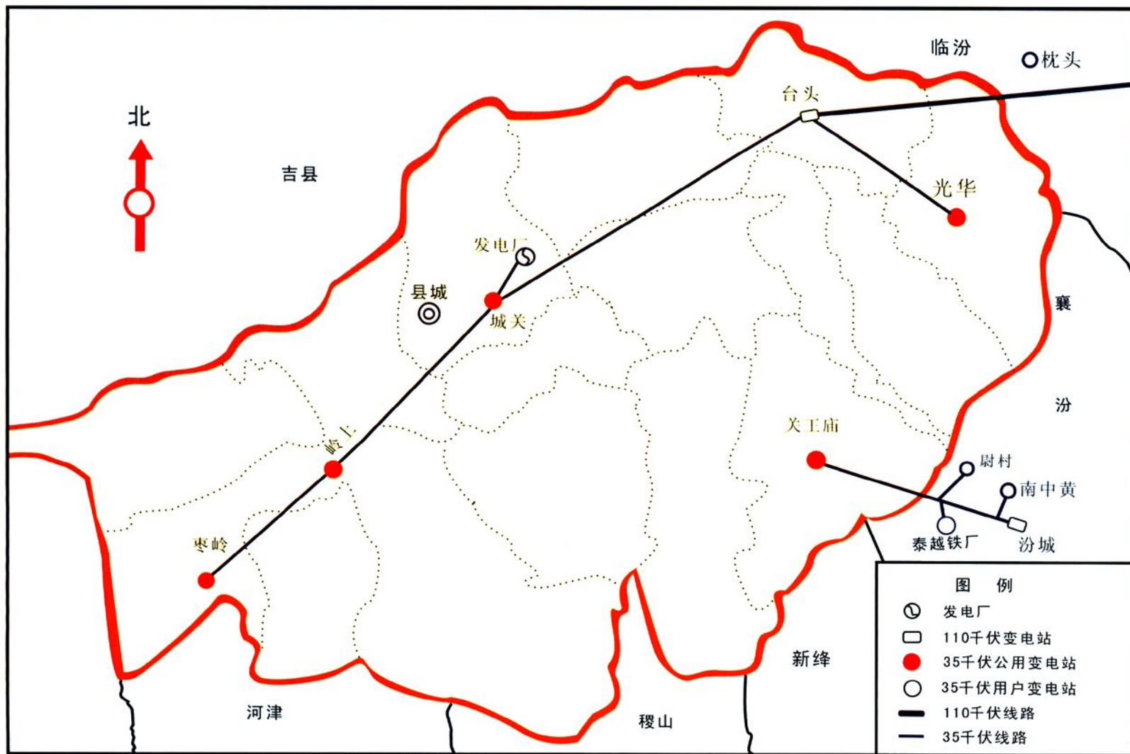
乡宁县电网地理接线示意图
