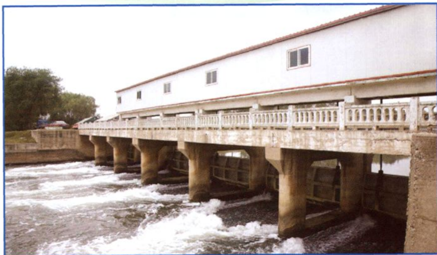
滦河下游灌区孟营节制闸
