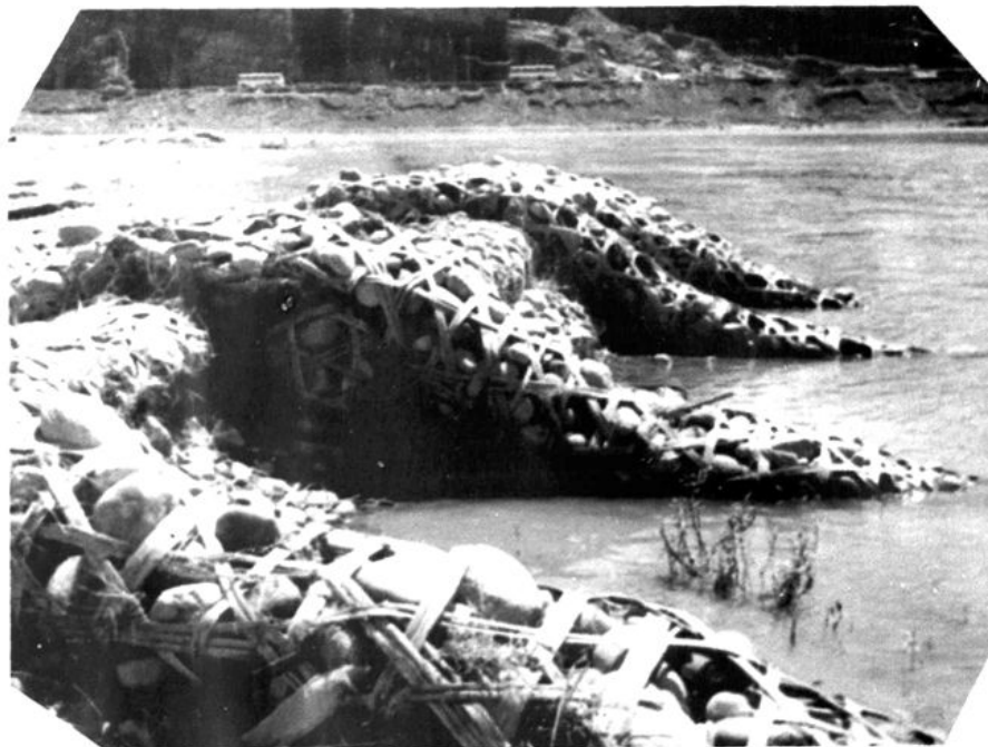
通济堰从古至今使用的“竹笼垒石为堤”的卵石竹笼工程。
