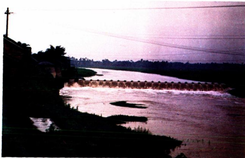
通济堰是一座多水源的引水灌区。图为拦截通济堰配水水量和体泉江水量入渠的体泉江拦河闸坝。
