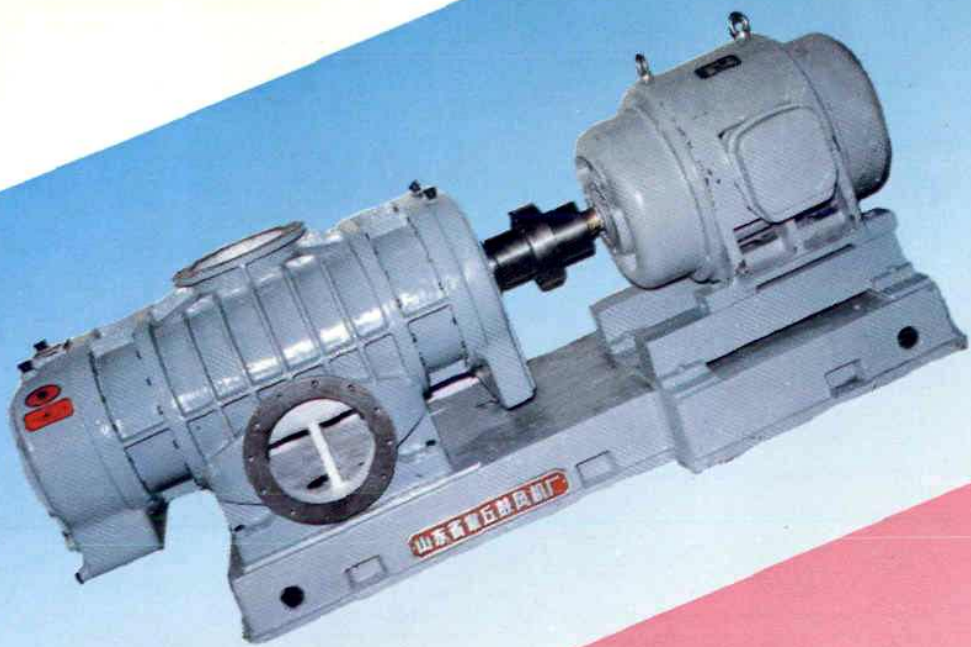
齐鲁牌LL74WD型罗茨鼓风机
