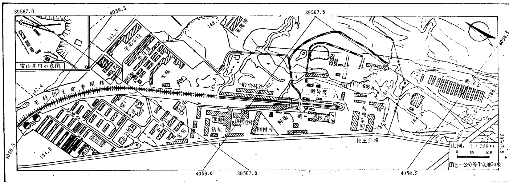
山东王村铝土矿平面图
