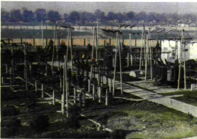
110KV 老河口变电站
