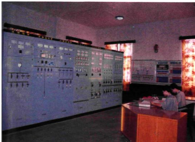
35KV 李楼变电站
