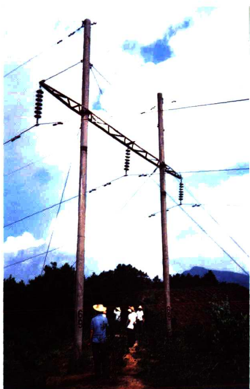
▲ 技术人员巡视110千伏输电线路
