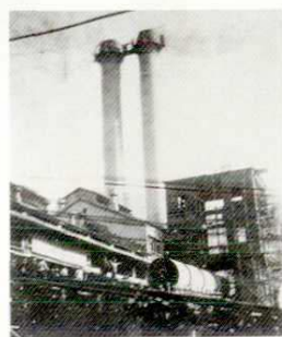
5号窑胴体吊装(1970年摄)
