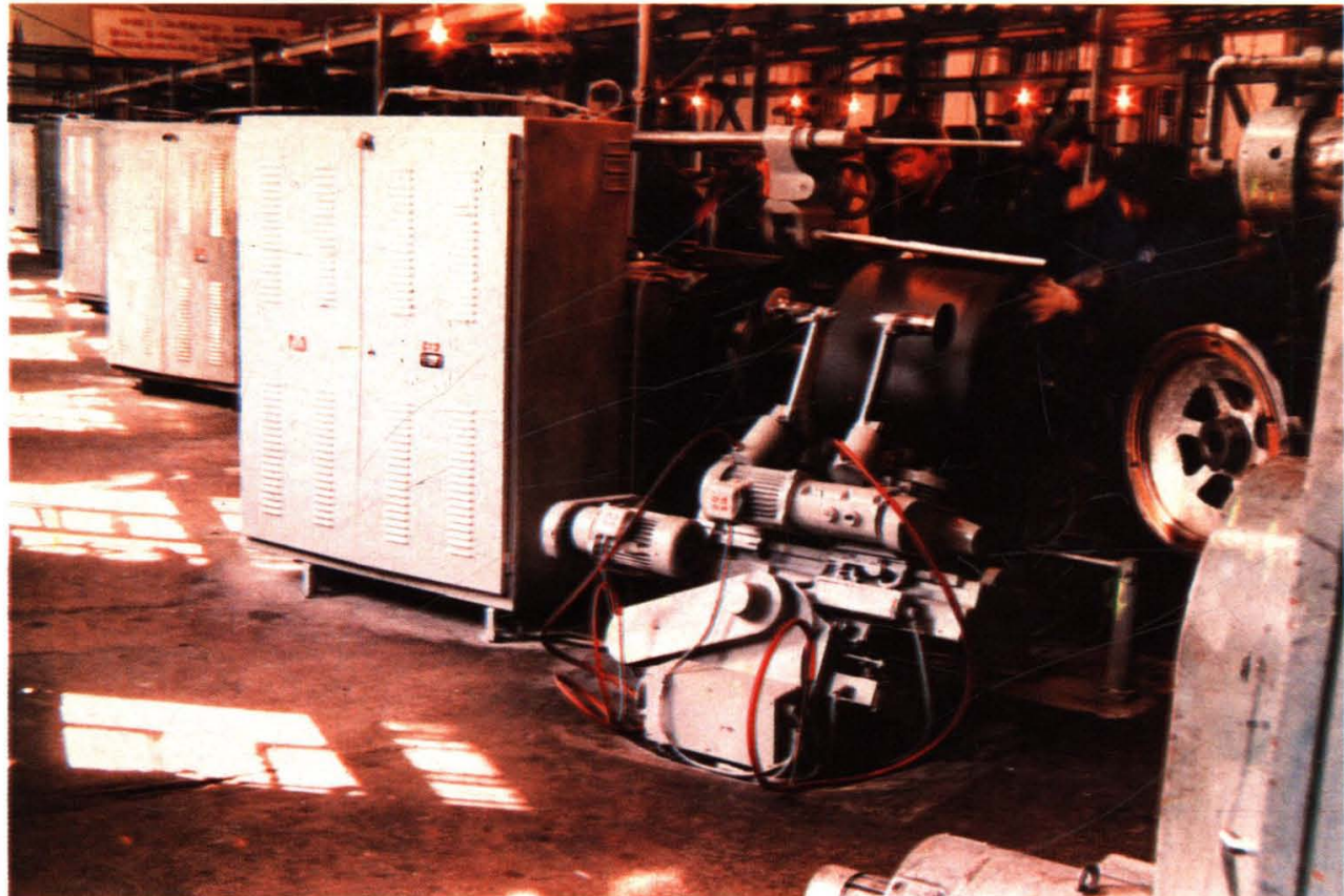
六十年代轮胎大会战中在牡丹江第一橡胶厂建立的外胎自动包边成型机群
