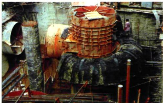
1998年12月，水轮机蜗壳安装
