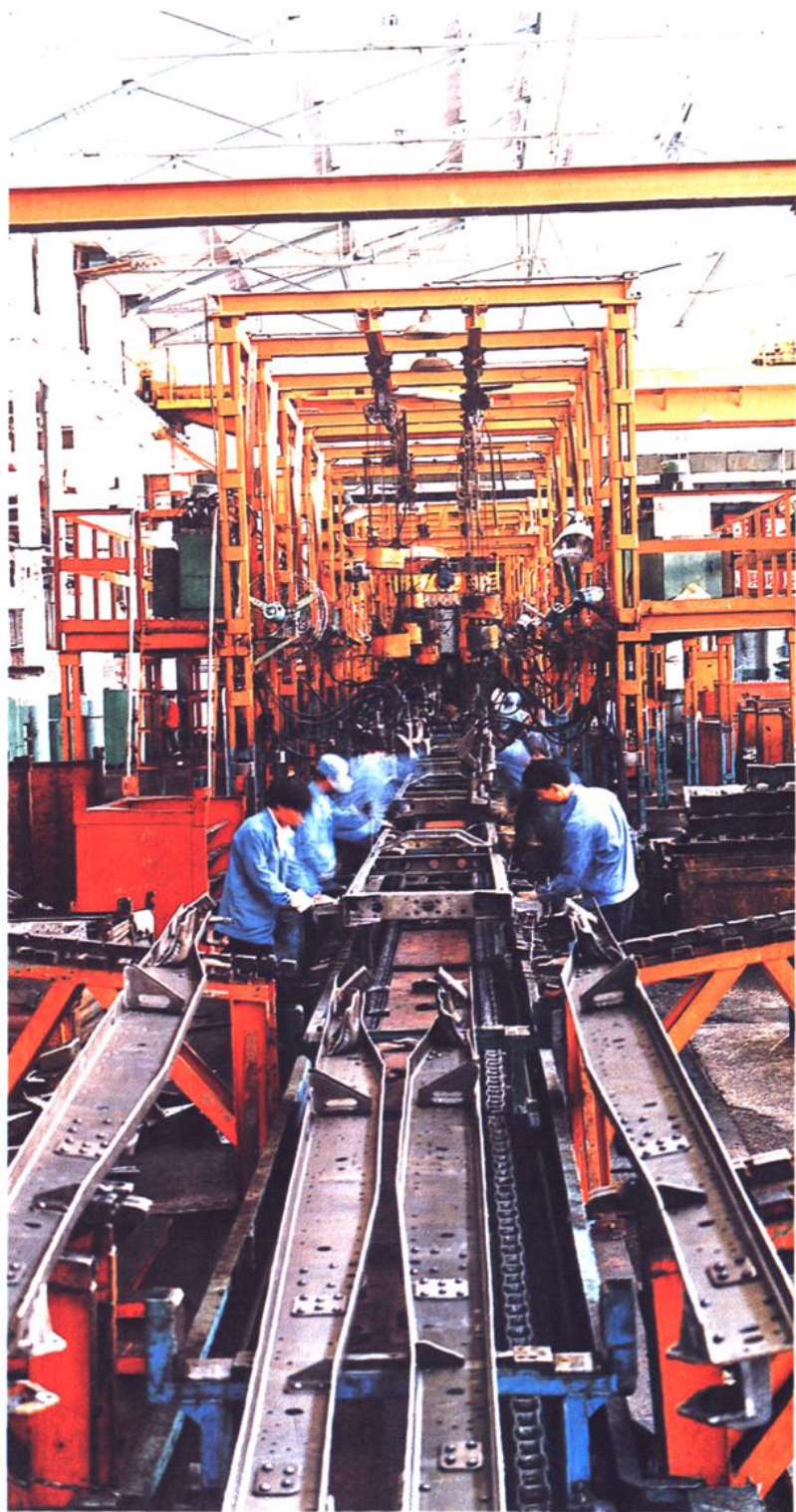
车架装配线
