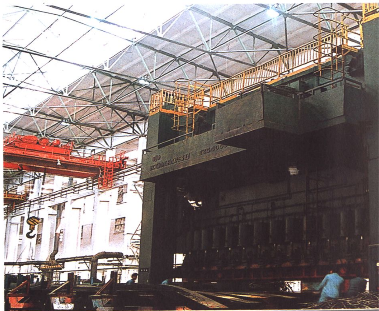
40兆牛压力机
