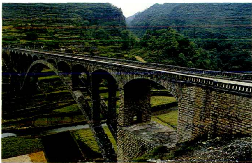
酃县红星双曲拱桥，主孔 107.36米
