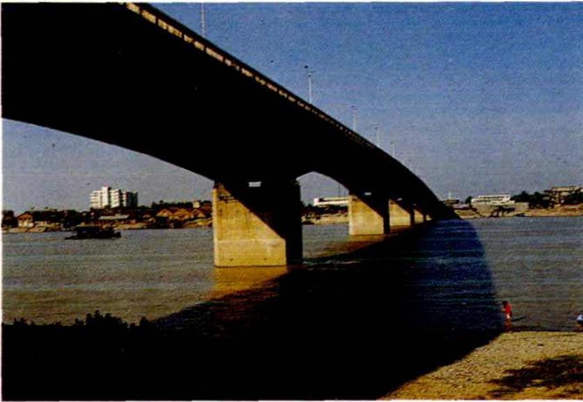
古丈县罗依溪双曲拱桥，主孔 116米，全长365米
