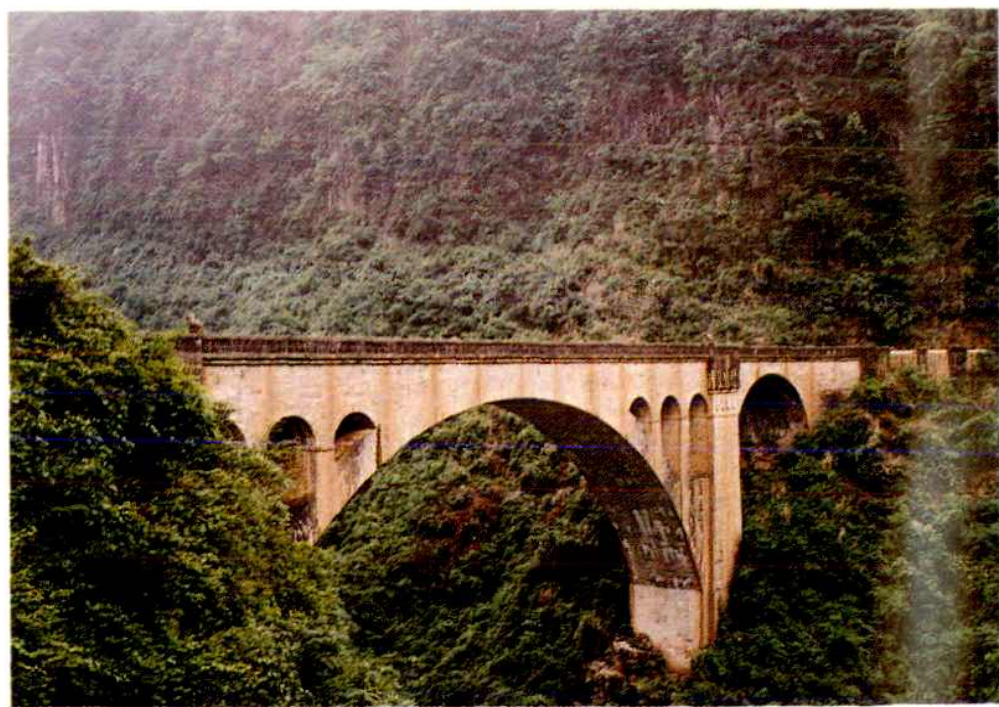
石门县黄虎港桥1959年建成，主孔60米突破 我国1300余年石拱桥跨径纪录
