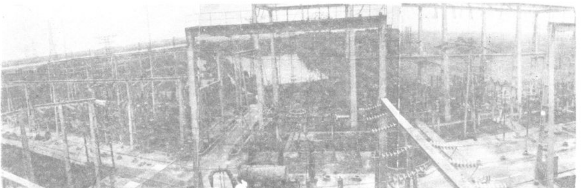
武圣宫 220 千伏变电站
