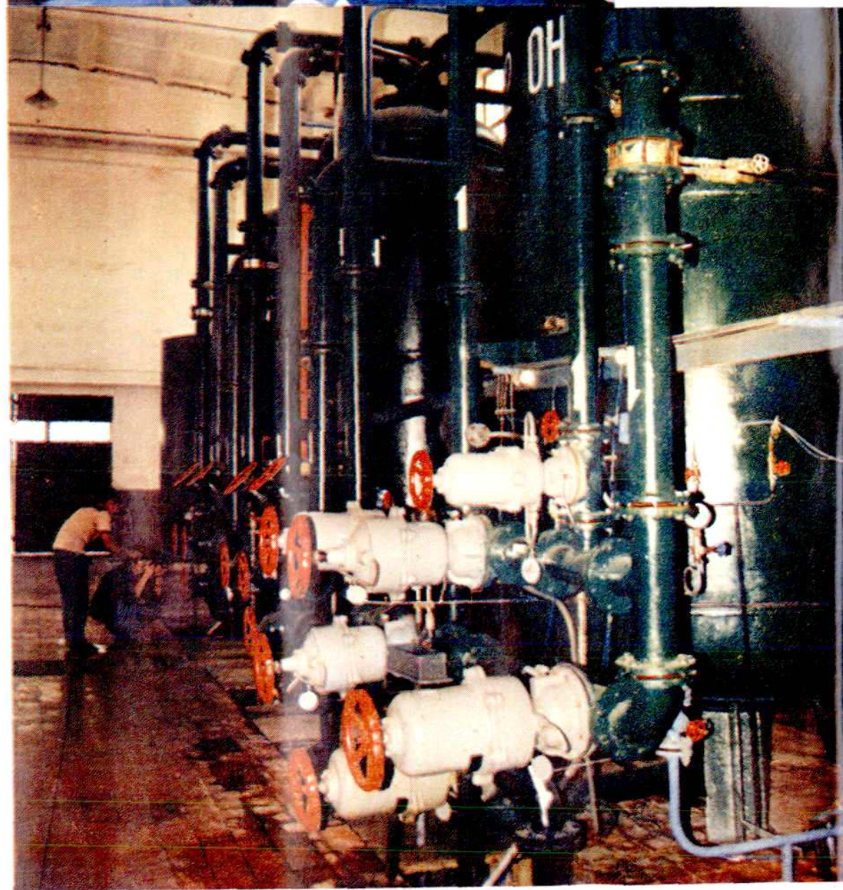
二电厂化学水处理室
