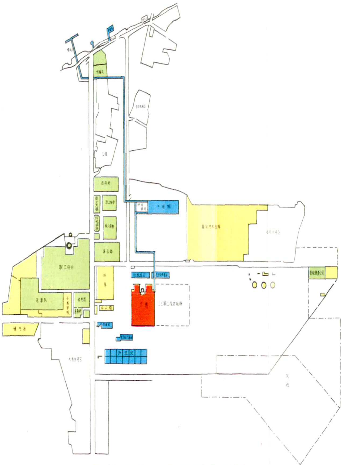
九江第二发电厂平面布置图
