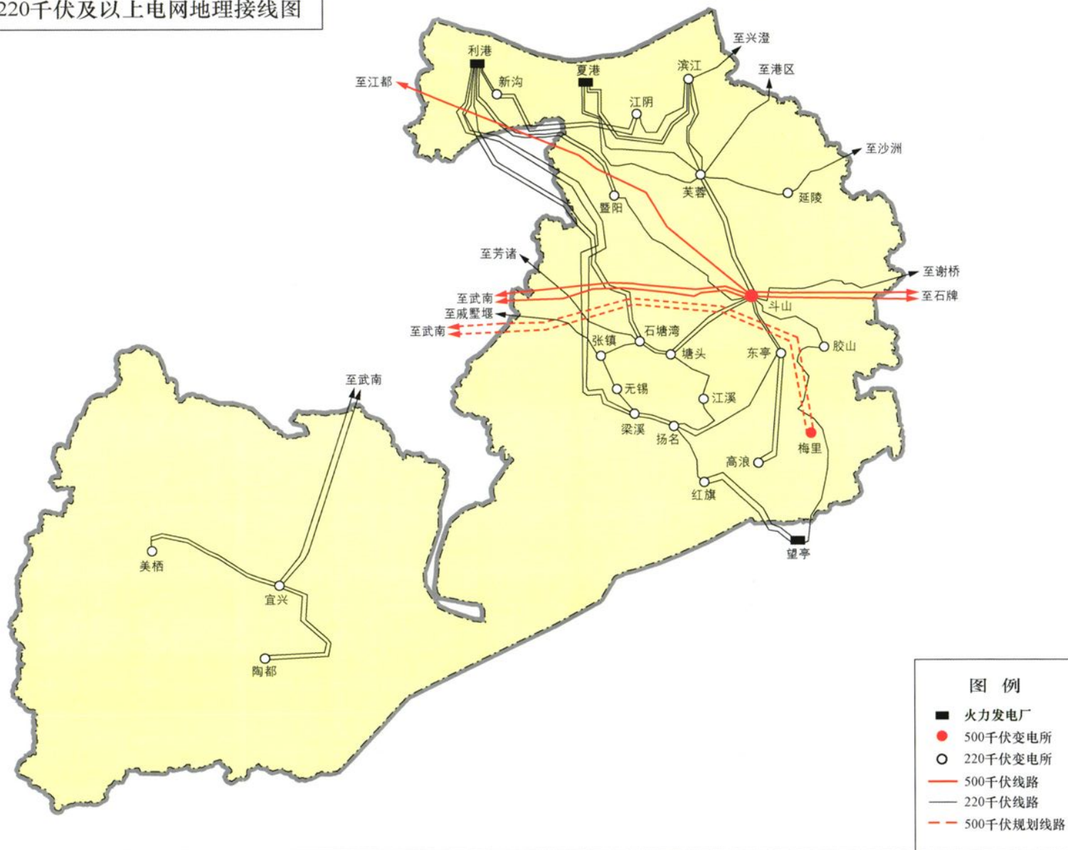
2002年无锡市220千伏及以上电网地理接线图
