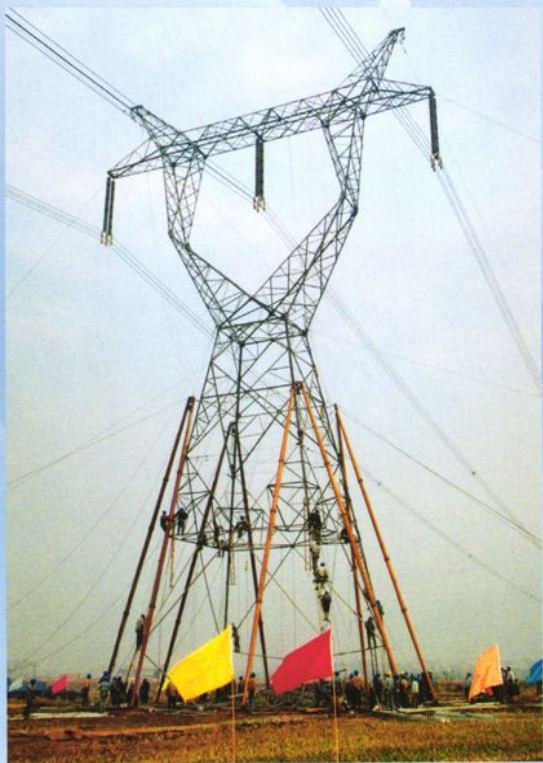
500千伏繁斗线650号塔带电平移35米、升高6米施工现场(1997年摄)
