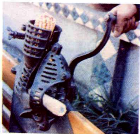
▲手摇式玉米脱粒机
