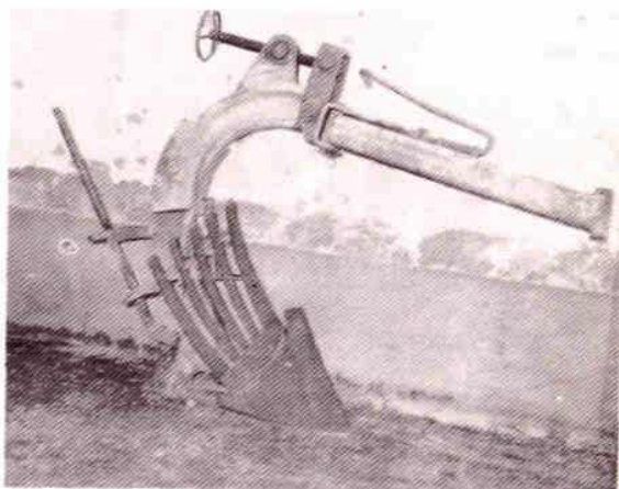
▲翻转犁
