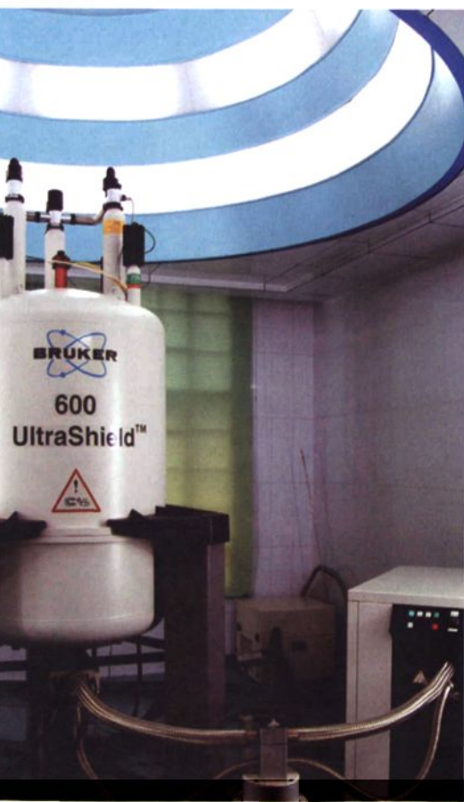
▲ 600兆超导超屏蔽傅立叶变换核磁共振波谱仪
